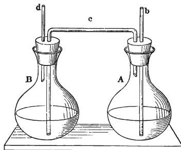
Фиг. 1. Алкалиметръ.
