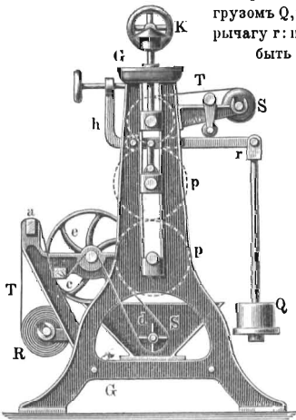
Рис. 8. Шлихтовальная машина.
