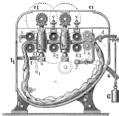
Рис. 12. Валицовая валильная машина.
