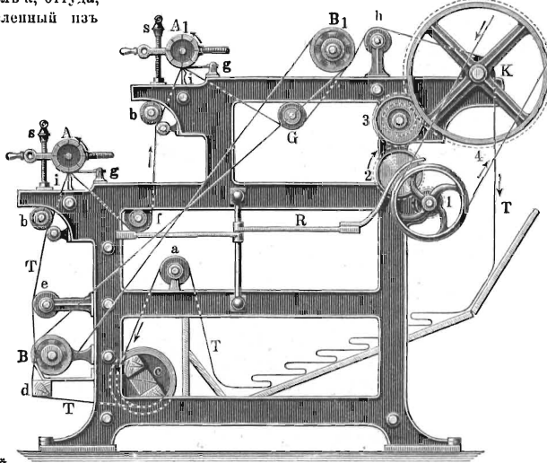
Рис. 5. Стригальная машина.
