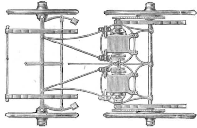
7. Повозочный стаягъ и 8. расположеиіе движущаго механизма коляски фирмы „American Vehicle Co.“
