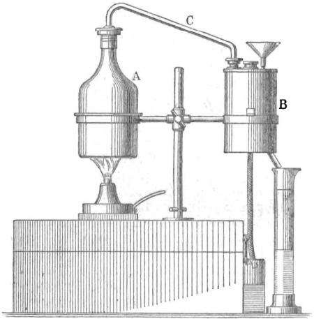
Фиг. 1. Перегонный аппаратъ для алкоголя.
