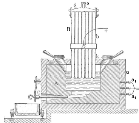
Фиг. 3. Аппаратъ Héroult для добыванія алюминія.
