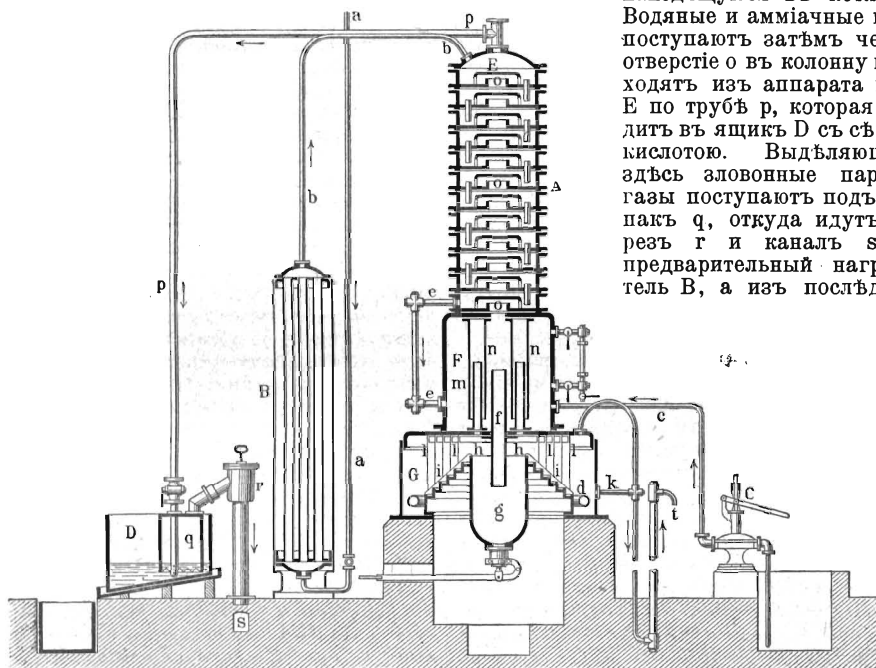
Аппаратъ Грюнеберга для получения нашатырнаго спирта и сѣрноокислаго амміака.
