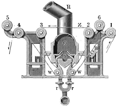
Рис. 3. Опальная (пальильная) машины.
