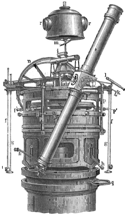
Альтазимуть Страсбургской обсерватории.
