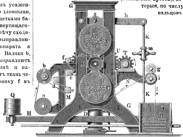
Рис. 9. Гладильная машина.
