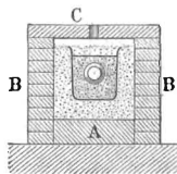
Фиг. 1. Продольный разрѣзъ. Аппаратъ Cowles для добыванія алюминія.
