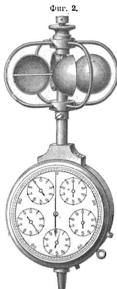
Анемометръ Робинзона.
