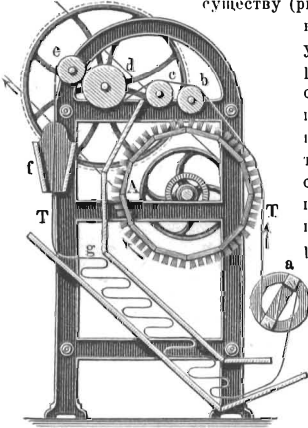
Рис. 7. Чесальная машина.
