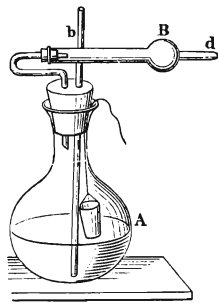
Фиг. 2. Ацидиметръ.
