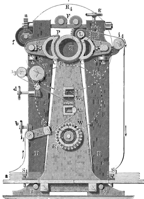
Рис. 10. Гладильная машина.
