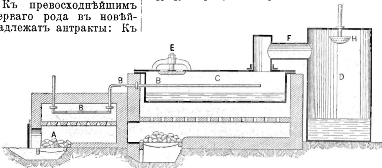
Аппаратъ для добыванія антрацена.
