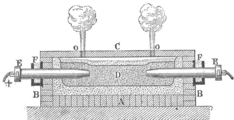
Фиг. 1. Продольный разрѣзъ. Аппаратъ Cowles для добыванія алюминія.
