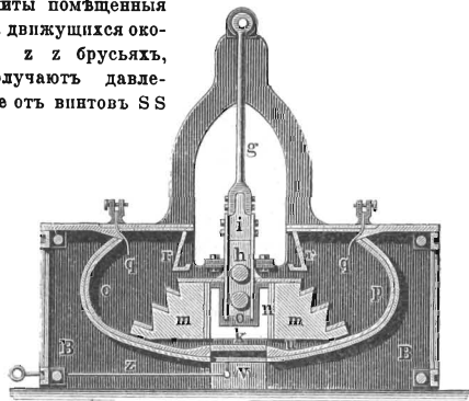
Рис. 11. Валильная машина.
