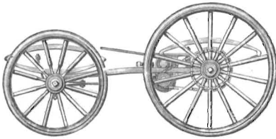
7. Повозочный стаягъ и 8. расположеиіе движущаго механизма коляски фирмы „American Vehicle Co.“
