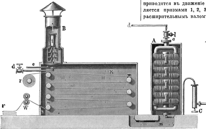
Рис. 1. Сушильная камера.
