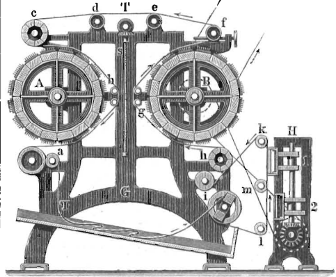
Рис. 6. Ворсовая (ворсовальная) машина.
