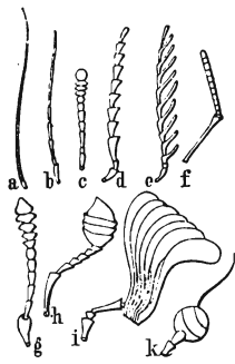
Антенны насекомыхъ.
