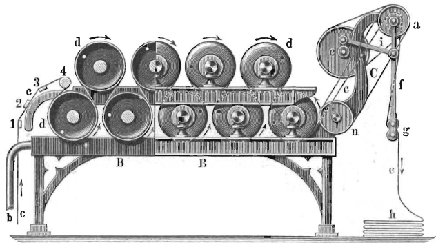
Рис. 2. Барабанная сушильная машина.
