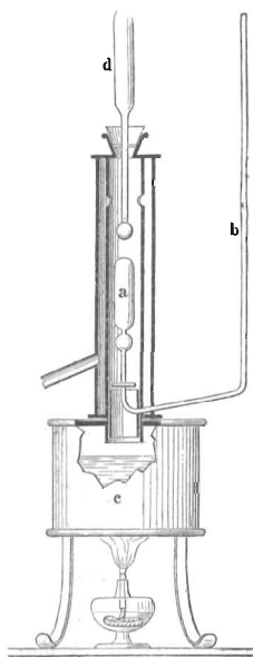
Фиг. 2. Вапориметръ.
