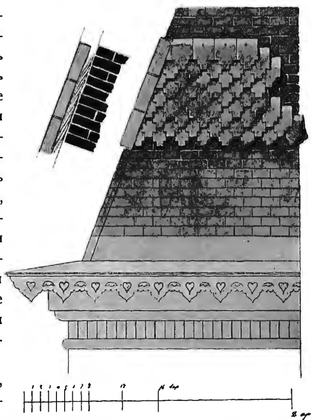
Рис. III. Черепица и подзоры на верхахъ кремлевскихъ башенъ.
