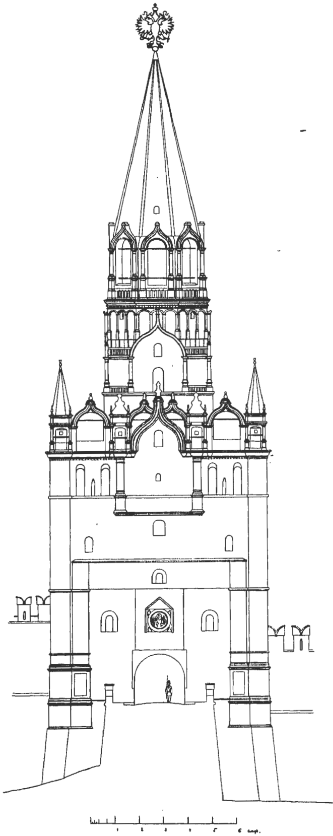
Рис. 169. Лицевой фасадъ Троицкой башни.
