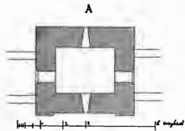
Рис. 304. 3-й этажъ.
