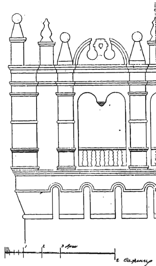
Рис. 182. Архитектурная обработка верха Кутафьи.
