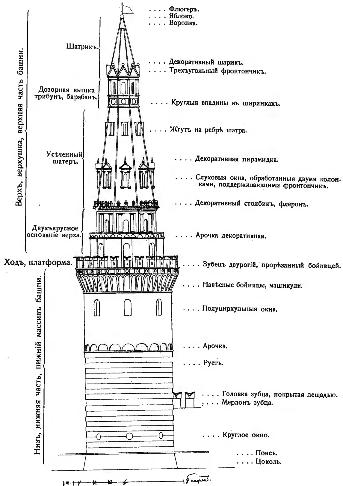
Рис. 114. Названія архитектурныхъ частей башенъ.
