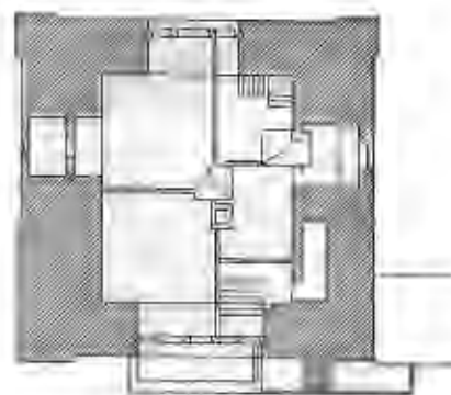
Рис. 273. 2-й этажъ.
