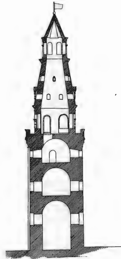
Рис. 303. Разрѣзь по линіи А В.
