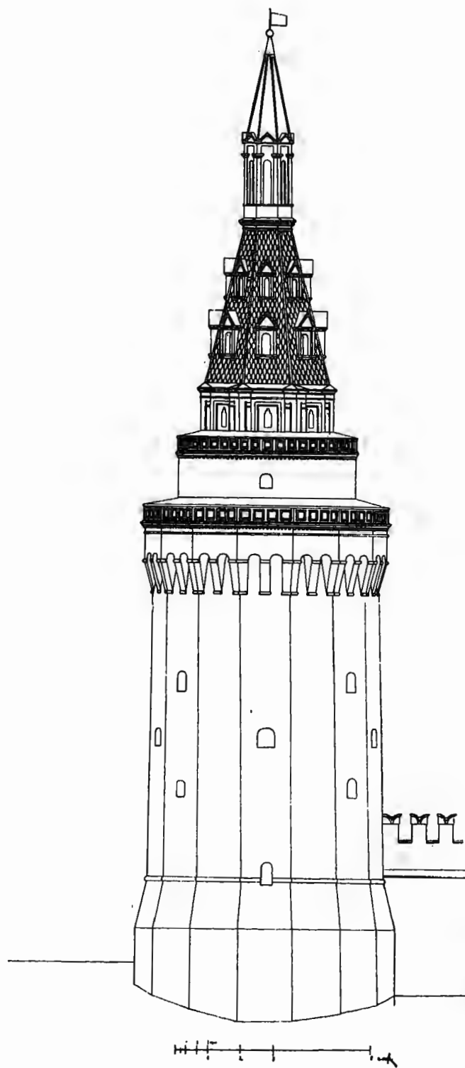
Рис. 260. Фасадъ со стороны 1-го Кремлевскаго Сада.
