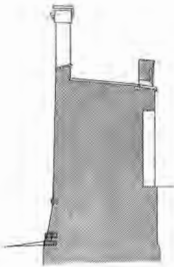
Рис. 85. Разрѣзъ стѣны между Тайницкой и Благовѣщенской башнями. [Масштабъ увелич. вдвое].
