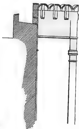
Рис. 89. Разрѣзь и изломъ стѣны между Оружейной и Боровицкой башнями.
