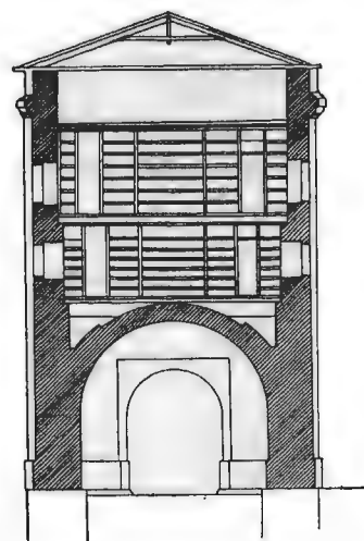
Рис. 188. Разрѣзъ отводной стрѣльницы.
