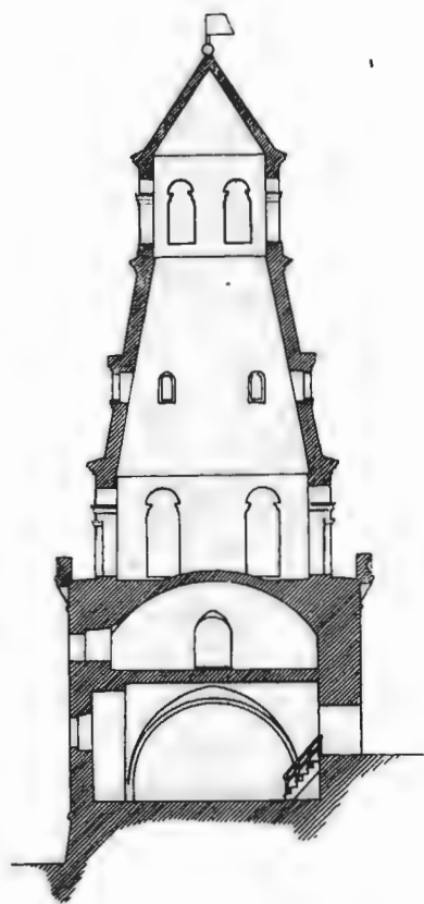
Рис. 325. Разрѣзь по линіи А В.
