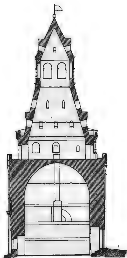
Рис. 271. Разрѣзь по линіи А. В.
