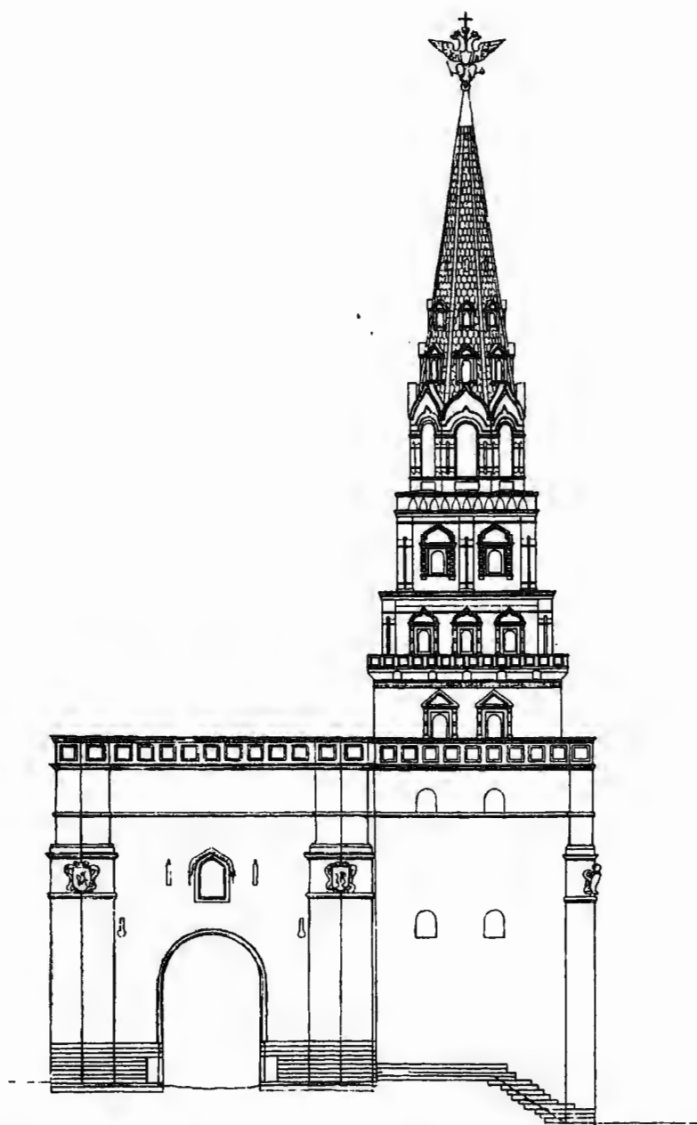
Рис. 202. Фасадъ Боровицкой башни со стороны Кремлевскаго сада.
