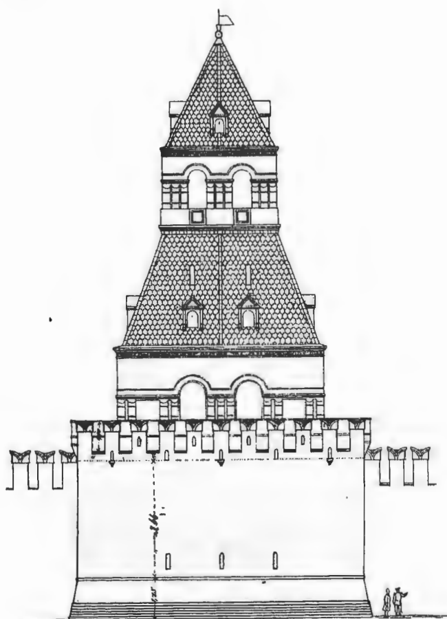
Рис. 226. Фасадъ Тайницкой башни со стороны Москвы рѣки.
