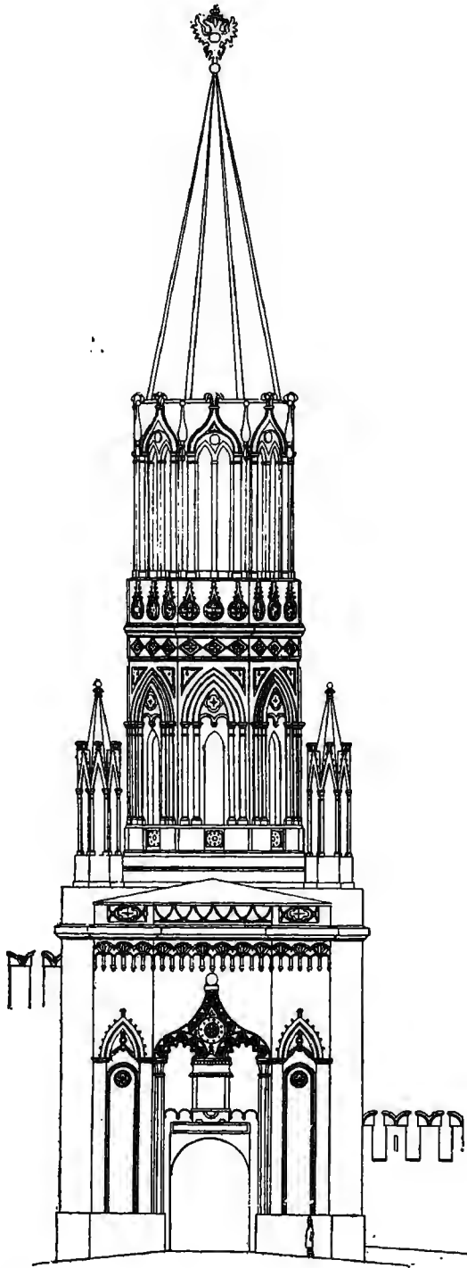
Рис. 186. Фасадъ со стороны Красной площади.
