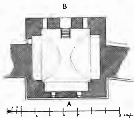
Рис. 326. 1-й этажъ.
