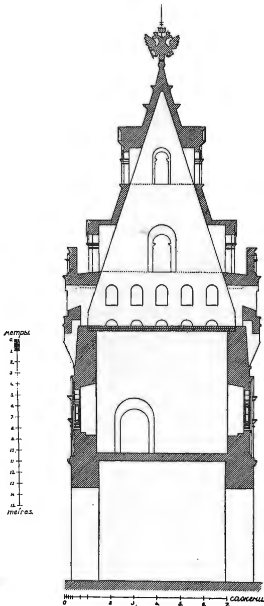
Рис. 72. Гербовая башня.
