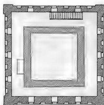
Рис. 125. 5-й этажъ.
