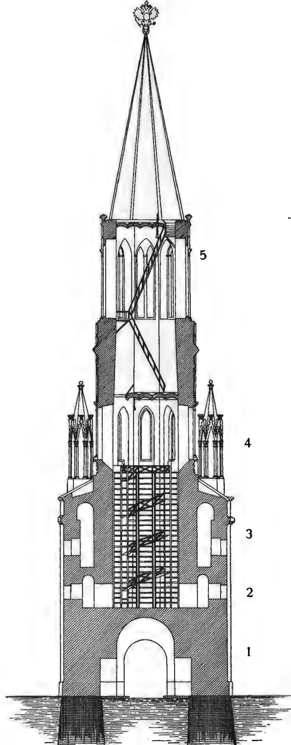
Рис. 187. Разрѣзъ по линіи А В.
