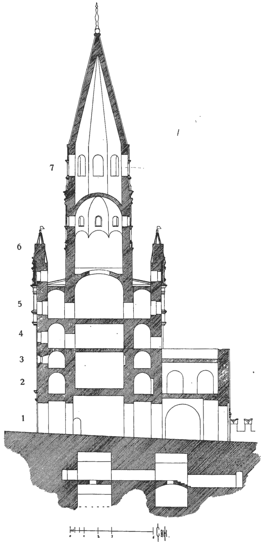
Рис. 170. Боковой разръзъ Троицкой башни.
