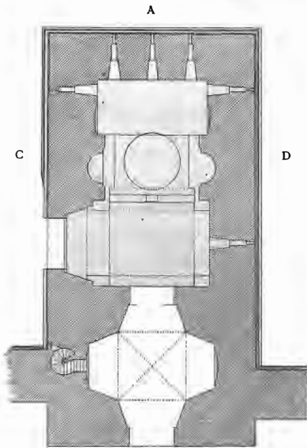
Рис. 230. 1-й этаж.
