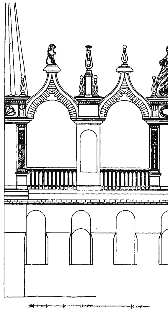
Рис. 134. 6-й этаж. Декоративная обработка боковых фасадов Спасской башни.
