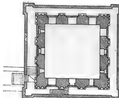
Рис. 275. 4-й этажъ.
