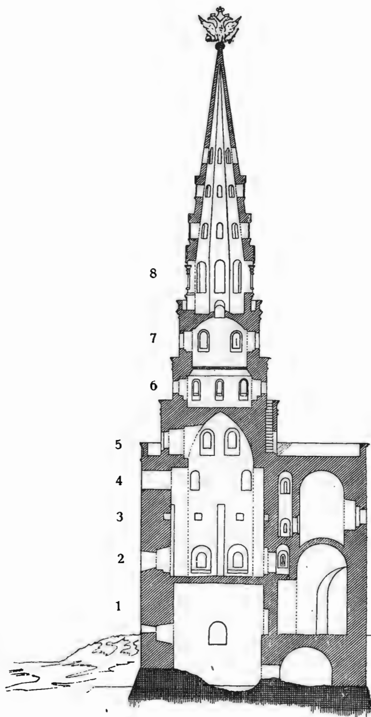
Рис. 203. Разрѣзь Боровицкой башни.
