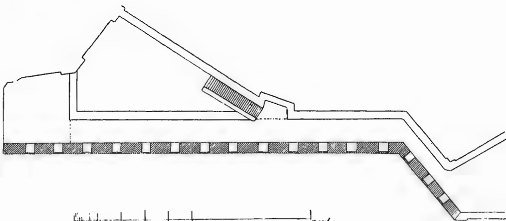
Рис. 87. Планъ стѣны между Оружейной и Боровицкой башнями. Фасадъ показаннаго на этомъ планѣ излома стѣны см. на рис. 89.
