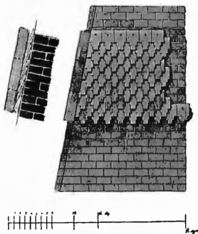
Рис. 113. Черепица на шатрахъ кремлевскихъ башенъ.
