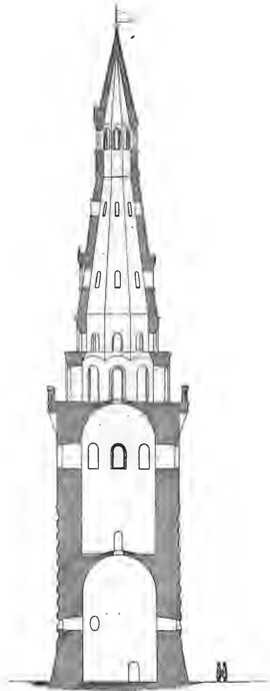
Рис. 252. Разрѣзь по линіи А В.
