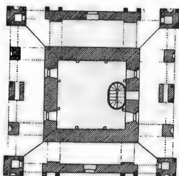
Рис. 127. 7-й этажъ.
