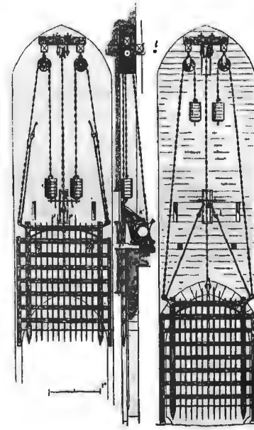
Рис. 38. Герсы въ Porte Narbo-naise въ г. Carcassone.
