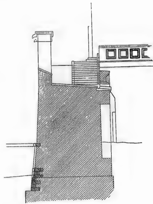
Рис. 86. Разрѣзъ стѣны между Благовѣщенской и Водовзводной башнями. [Масштабъ увелич. вдвое].
