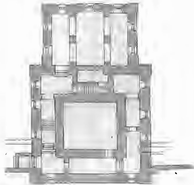
Рис. 174. 2-й этаж.
