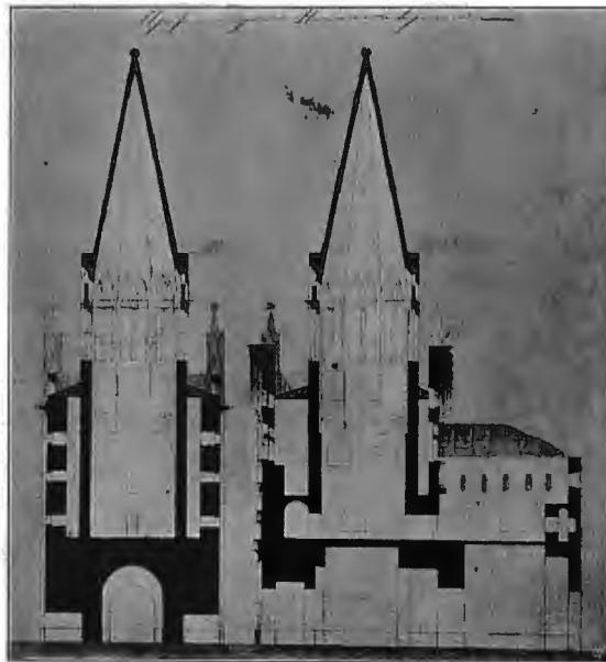
Рис. 197. Прямой и боковой разрѣзы Никольской башни, съ верхомъ, надстроеннымъ арх. Росси.
