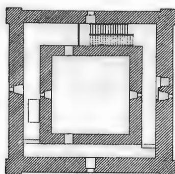
Рис. 124. 4-й этажъ.
