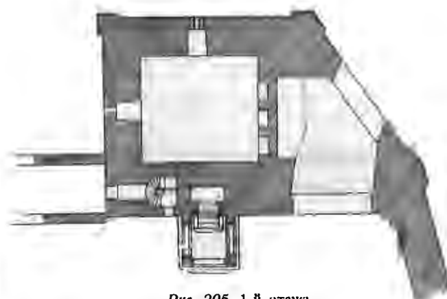
Рис. 205. 1-й этаж.
