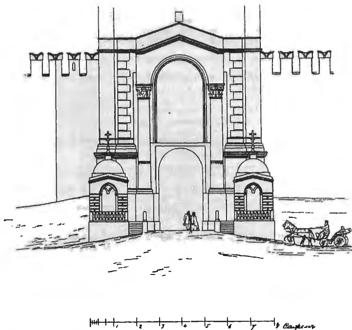
Рис. 165. Порталь Спасской башни и двѣ часовни, существовавшія до реставраціи 1866 года.
