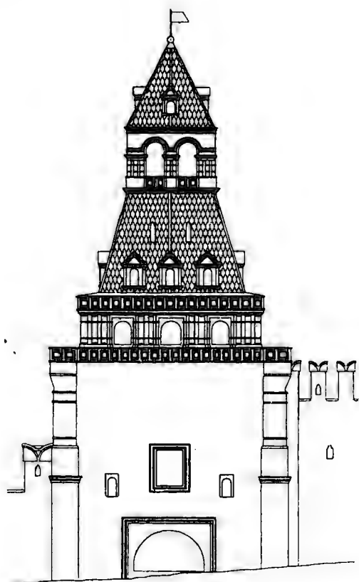
Рис. 270. Фасадъ со стороны Васильевской площади.
