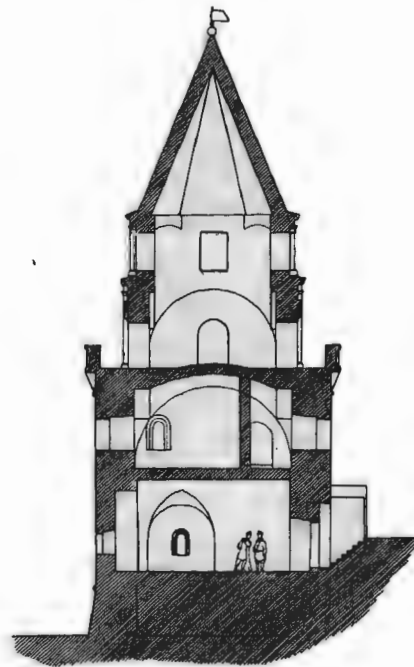
Рис. 347. Разрѣзь по линіи А В.
