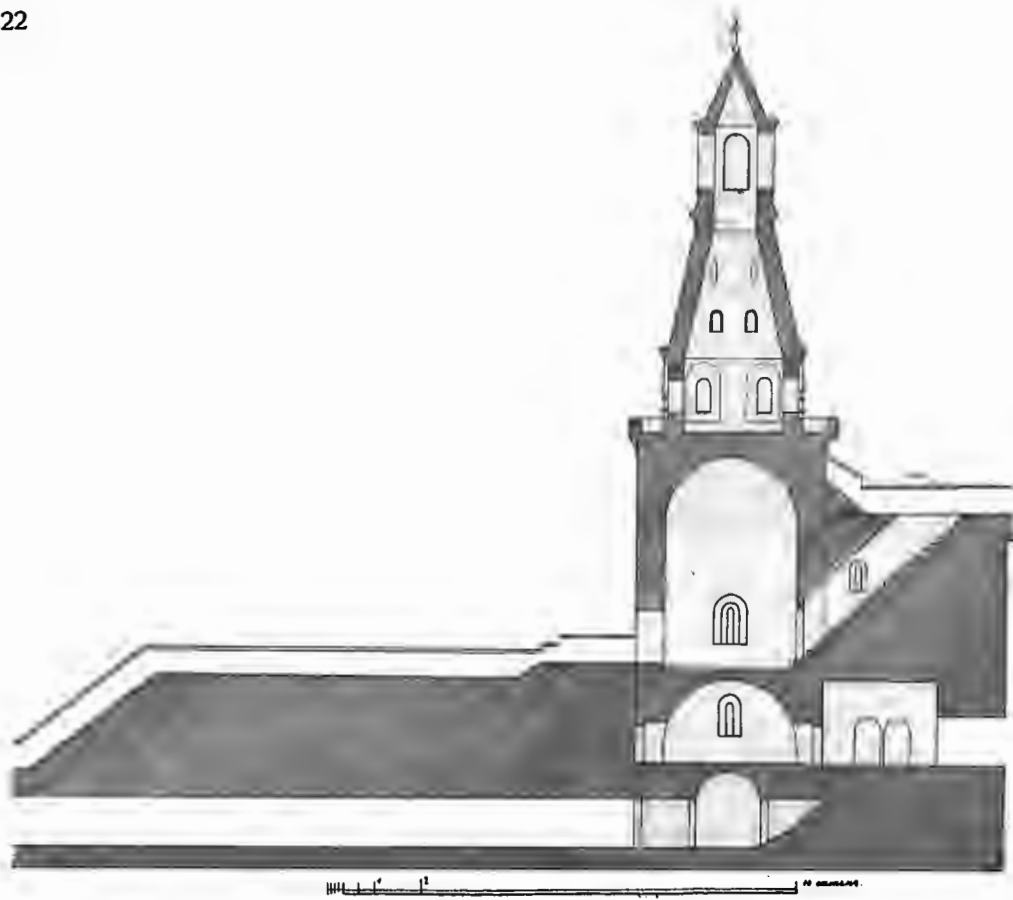
Рис. 285. Разрѣзъ Набатной башни и стѣны, къ ней прилегающей по линіи А В.
