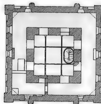
Рис. 126. 6-й этажъ.
