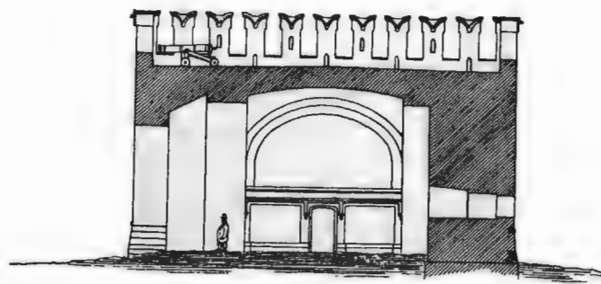
Рис. 228. Разрѣзь отводной башни по линіи С D.
