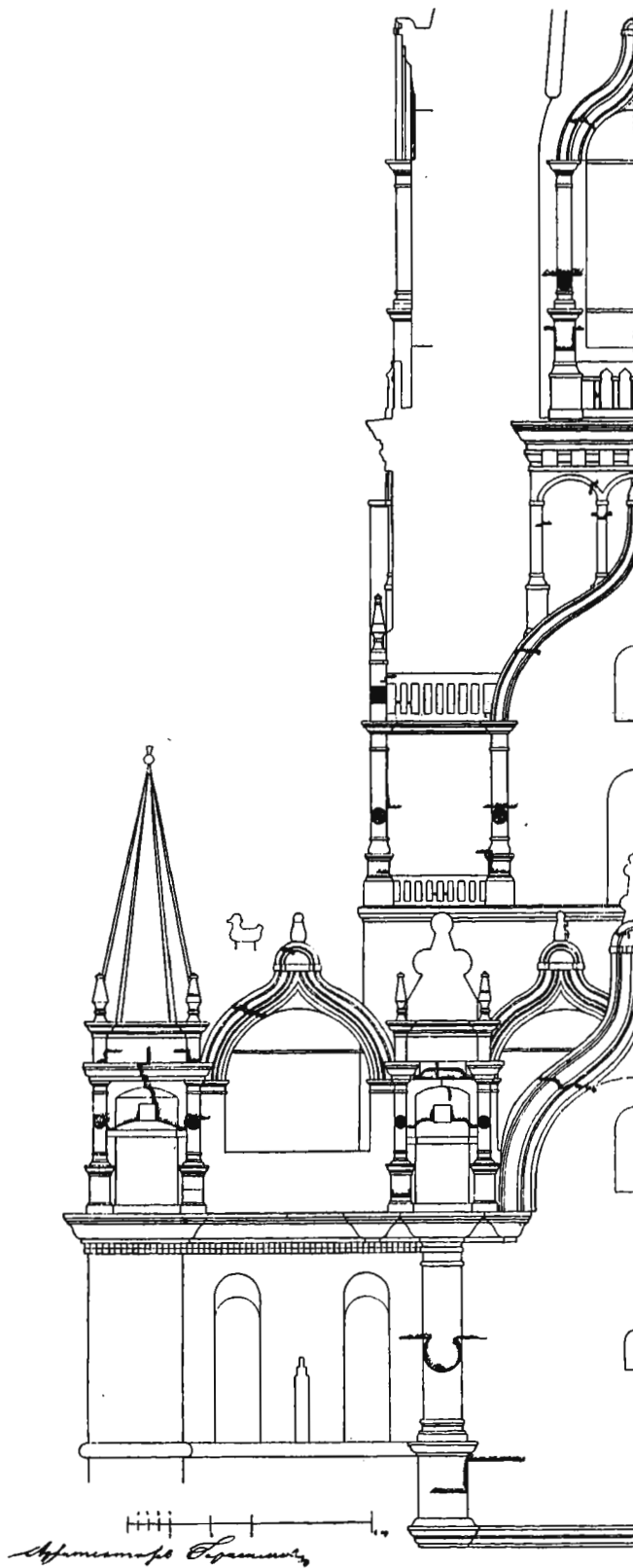
Рис. 179. Архитектурная обработка верха Троицкой башни.
