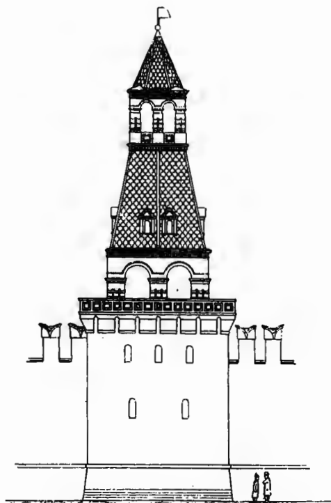
Рис. 333. Фасадъ со стороны Москвы рѣки.
