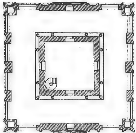
Рис. 177. 5-й этаж.
