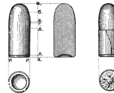
Рис.267. Пуля въ бумаж. обер.
