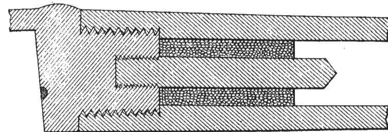
Рис. 10. Стержневой штуцер Тувенена.
