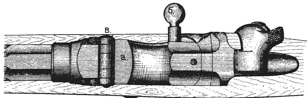
Рис.134. Видъ сверху.
