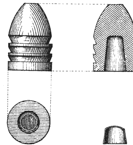
Рис. 13. Пуля Минье.
