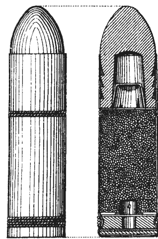
Боевой патронъ къ винтовкѣ Карле. Рис.131.
