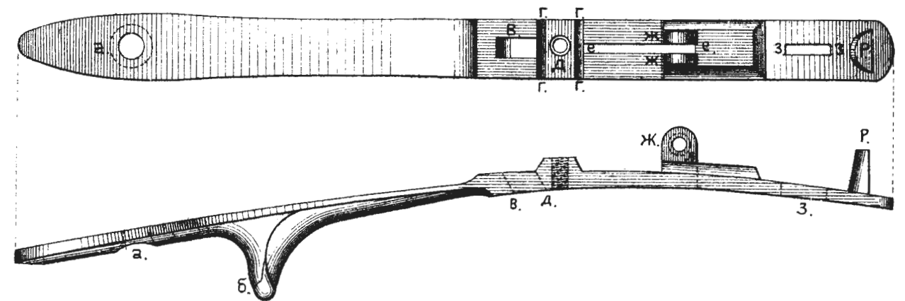
Рис.123. Спускъвая личинка.
