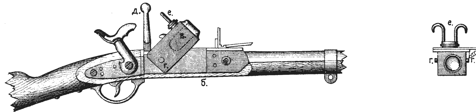
Рис.25. Ударное крепостное ружье обр.1839 г.
