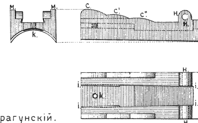
Рис.201. Прицѣльная колодка
