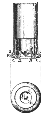
Рис.266. Просальникъ
