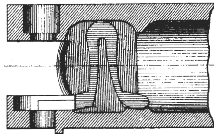
Рис.186. Положеніе отметной пружины.
