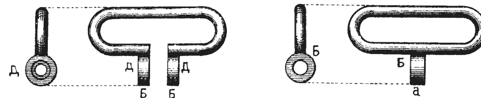
Рис.125. Нижн. антабка. Верхн. антабка.
