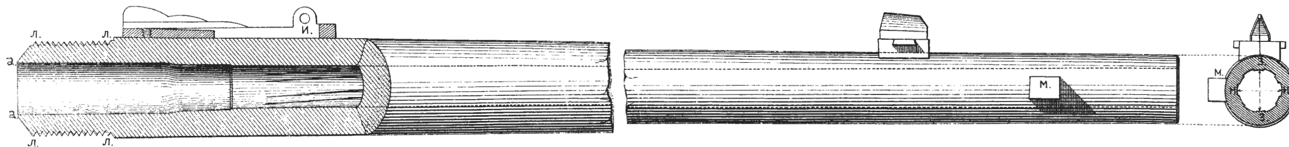
Рис.200. Ствол пѣхотной винтовки.
