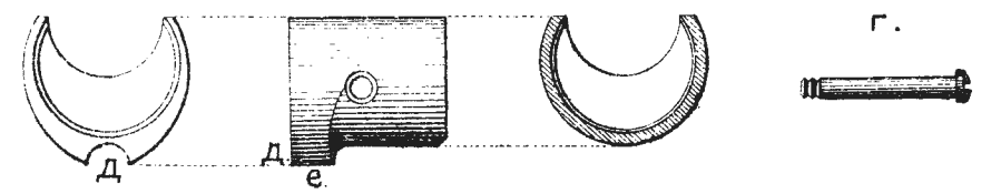
Рис. 240. Наконечникъ пѣхот. винтов.
