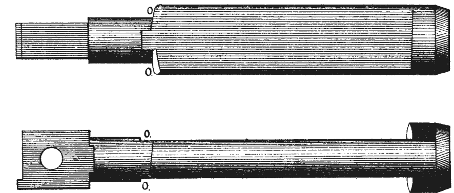
Рис.85. Стебель затвора.
