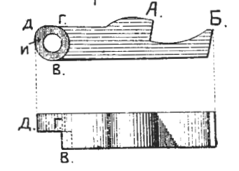
Рис.210.Затвор.задер.съ отражат.
