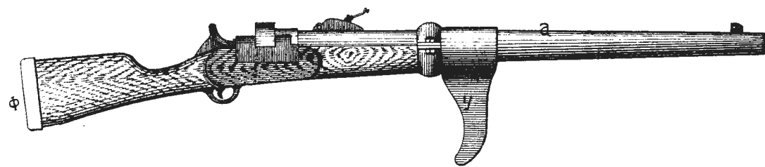
Рис.275. Замокъ къ кръпостному ружью образ.1876 г.
