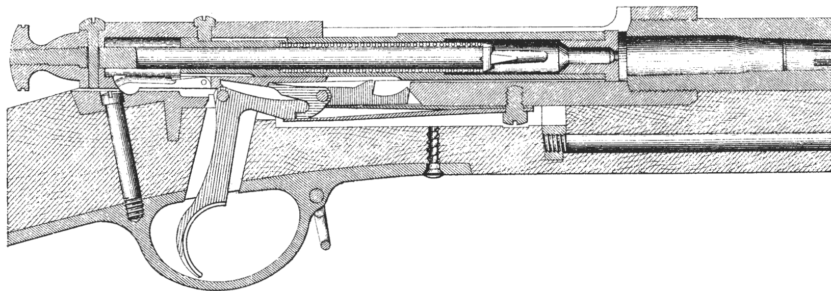
Рис.261. На предохранител. взводѣ.
