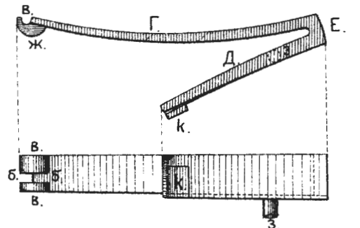
Рис.158.Боевая пружина.
