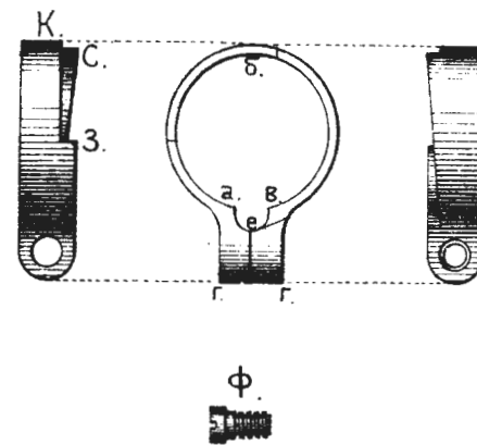
Рис.119. Хомутикъ.
