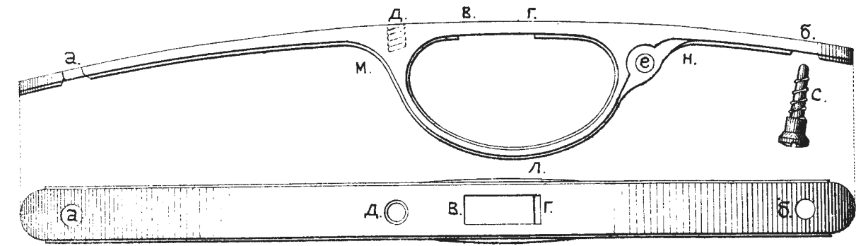
Рис. 242. Хвост. винтъ пѣхотной винтовки.
