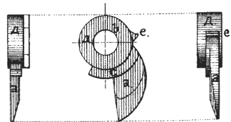
Рис.184. Выбрасыватель.
