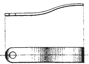
Рис.176. Подстрѣлочная пружина.
