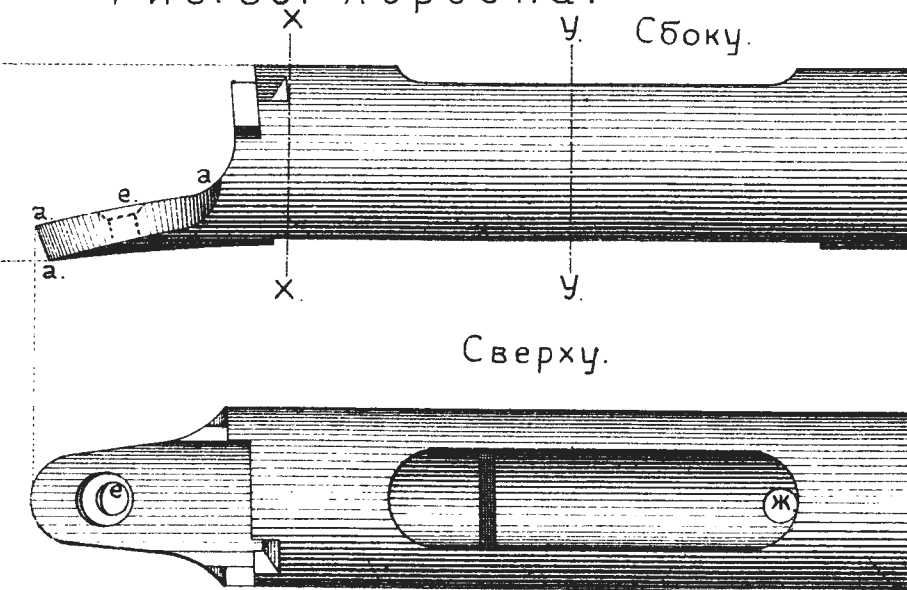
Рис. 89. Коробка.
