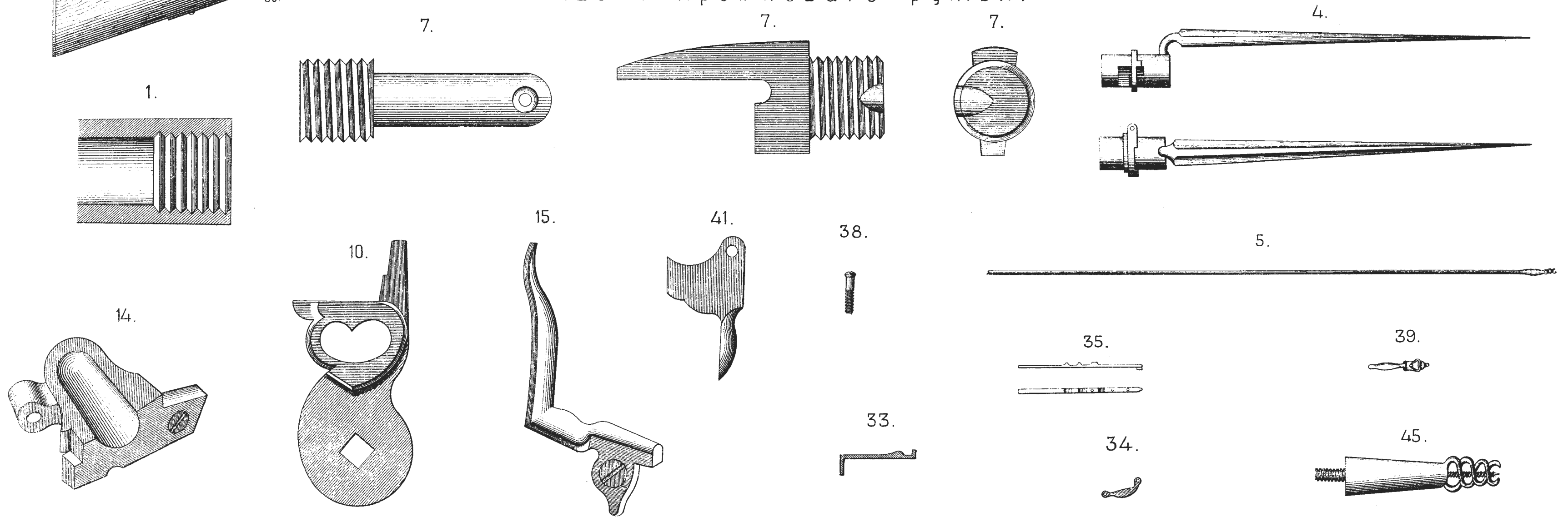
Рис. 2. Части Кремневого ружья.
