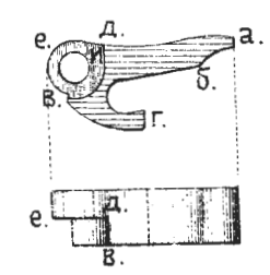
Рис.209.Крючекъ.
