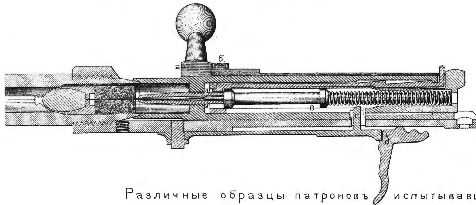
Рис. 60. Винтовка системы Дрейзе.
