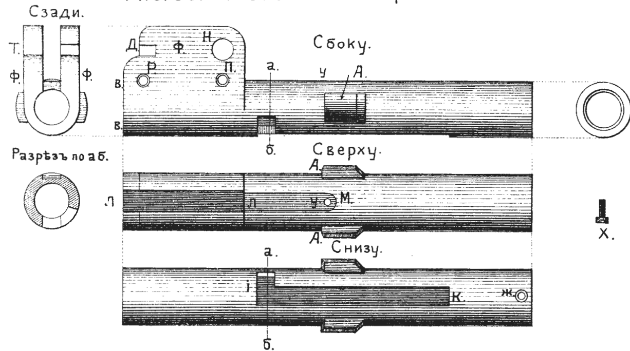
Рис. 96. Стебель затвора.
