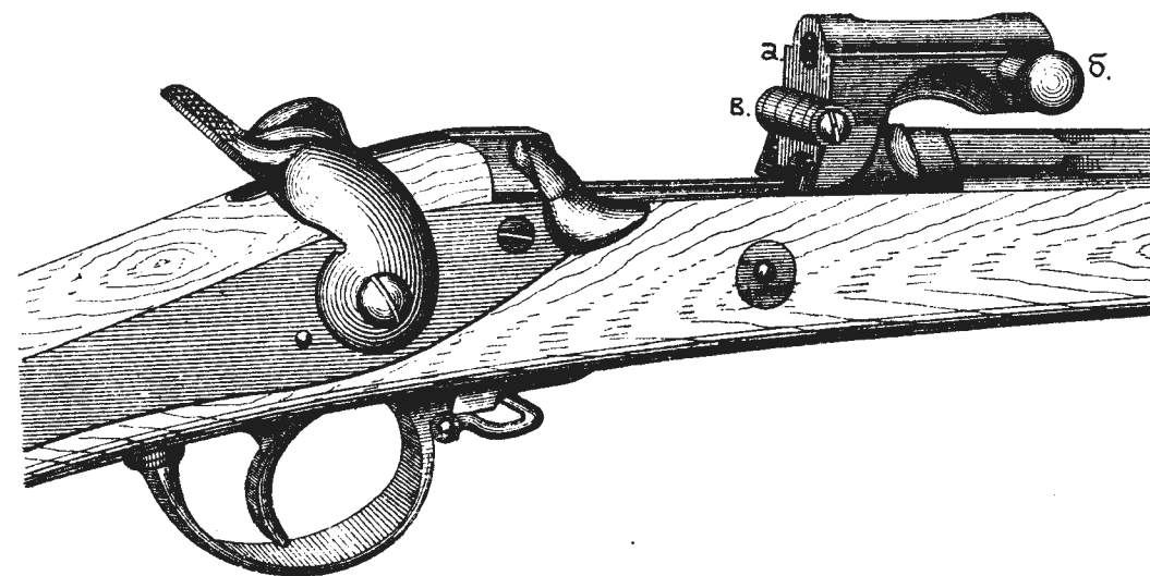
Рис.135. Затворъ открытъ.
