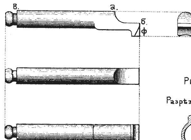
Рис.228. Выбрасыватель.
