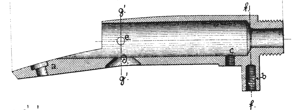
Рис.176. Подстрѣлочная пружина.
