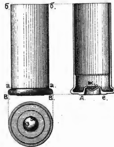
Рис.165. Гильза
