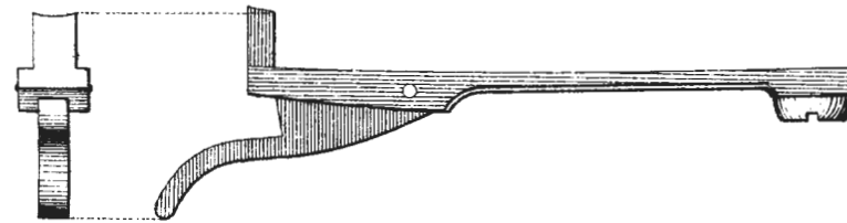
Рис. 91. Крючковая пружина.
