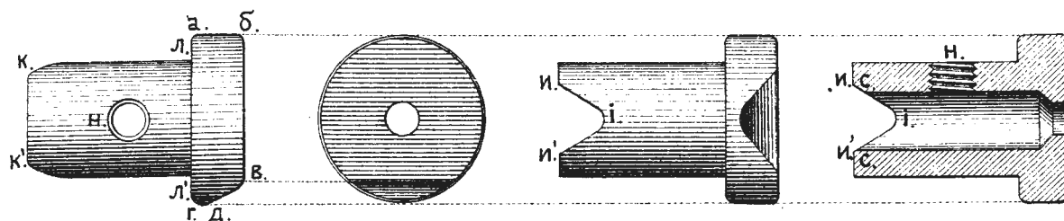
Рис.224. Винтъ боев. личинки.
