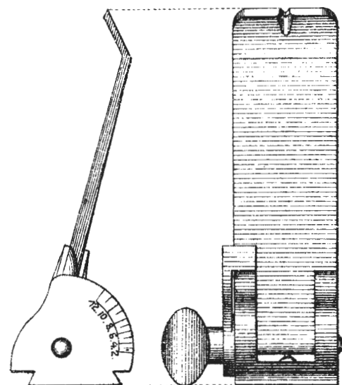
Рис. 111. Прицѣль въ собранномъ видѣ.
