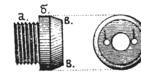
Рис. 97. Конусъ.
