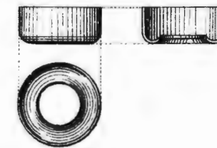
Рис.166. Мѣдная чашечка въ гильзу.
