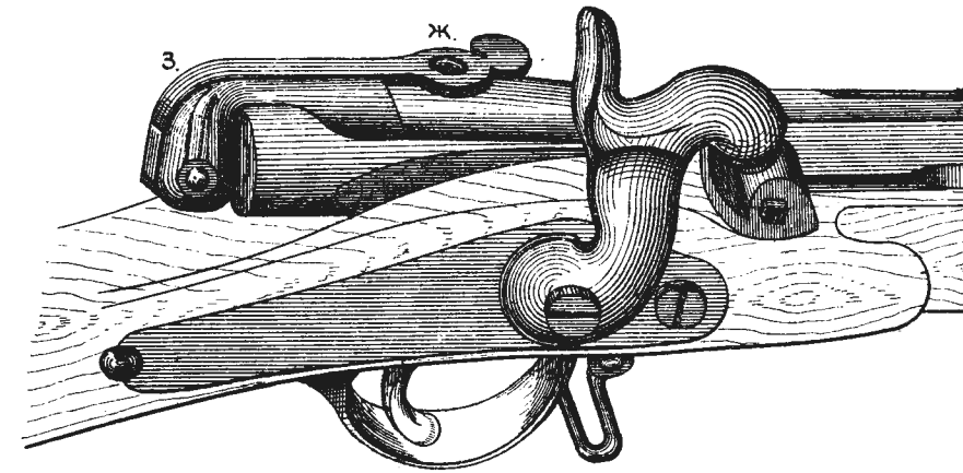
Рис.84. Затворъ закрытъ.
