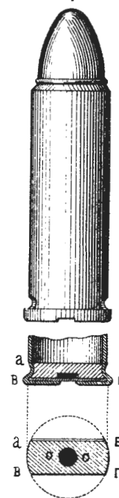
Рис. 73. Металлическій патронъ Мартини централн. воспламен.
