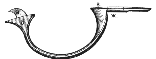
Рис.124. Скобочное колѣно.
