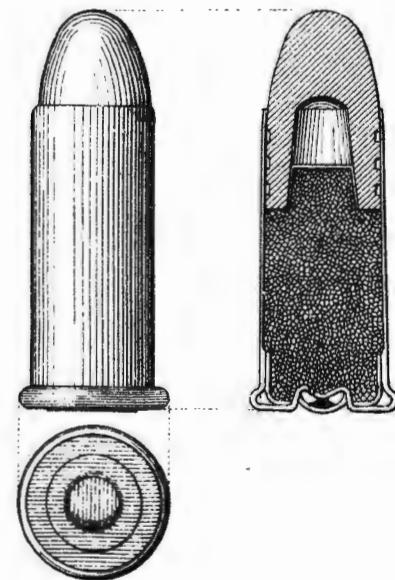
Рис.164. Патронъ къ винтовкѣ.
