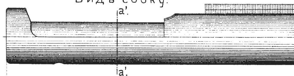
Рис.174. Ствольная коробка
