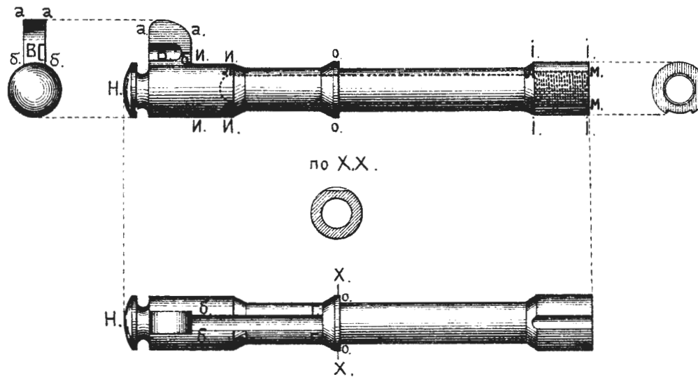
Рис. 104. Стебель ударника.
