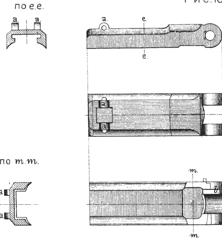
Рис.180. Стрѣлка.
