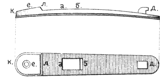
Рис.253. Спусков. личинка казачьей винтовки.
