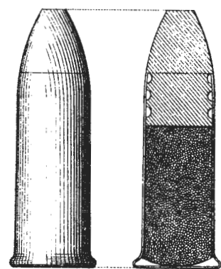
Рис. 72. Металлическій патронъ кругового воспламененія.
