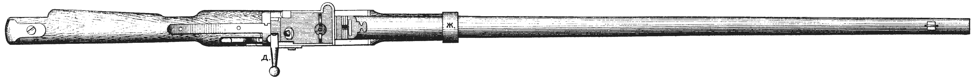
Рис.24. Ударное крепостное ружье обр.1839 г.
