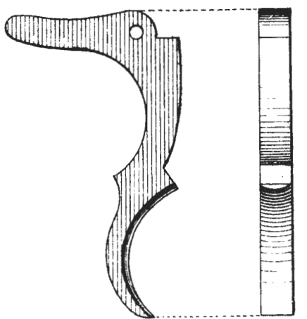
Рис.193. Спускъ.
