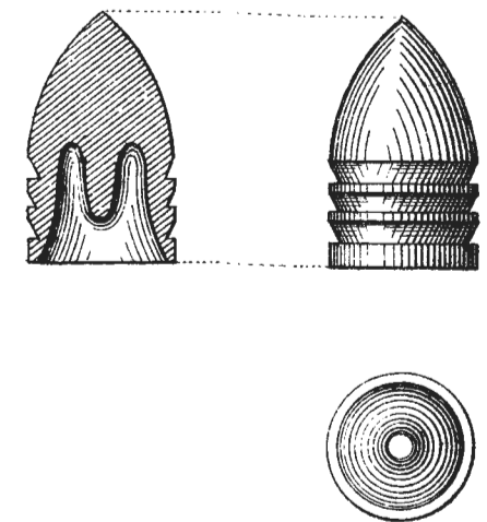
Рис. 15. Бельгійская пуля.
