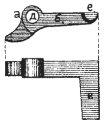
Рис.160.Крючекъ.
