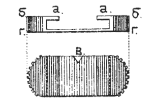
Рис.219.Боковой прицѣль.
