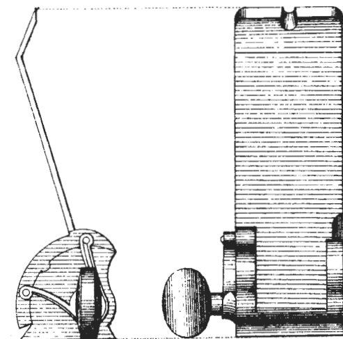
Рис.32. Гессенскій прицѣль Литтихск.штуцера.
