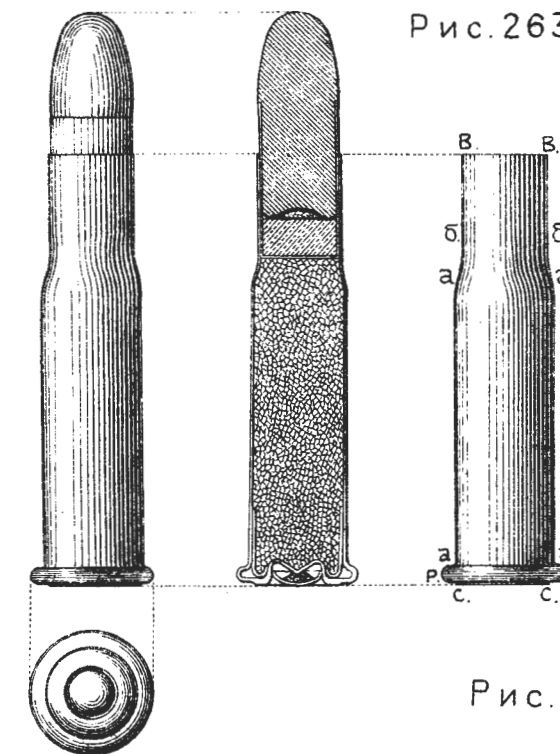
Рис.262. Боевой патр. къ винтовкѣ Бердана №2
