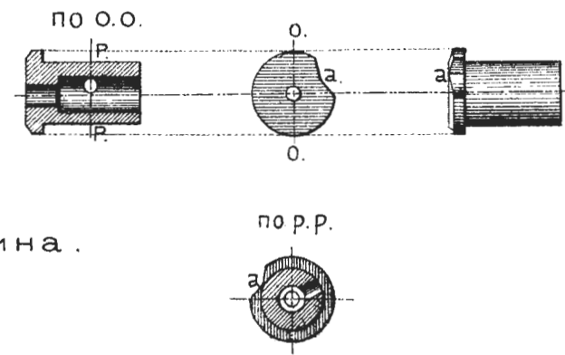
Рис.182. Личинка.
