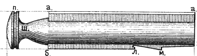
Рис.231. Замочная трубка.
