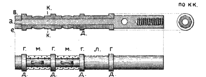
Рис.258. Протирка.
