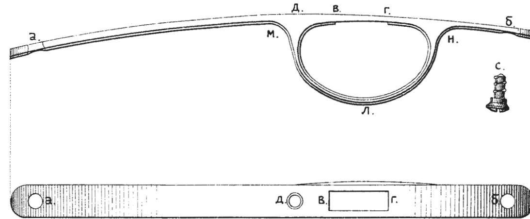
Рис.247. Спускная скоба драгунской винтовки.
