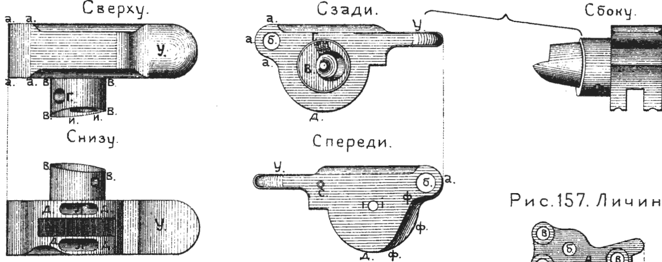
Рис.148.Затворъ съ бойкомъ и ударникомъ.
