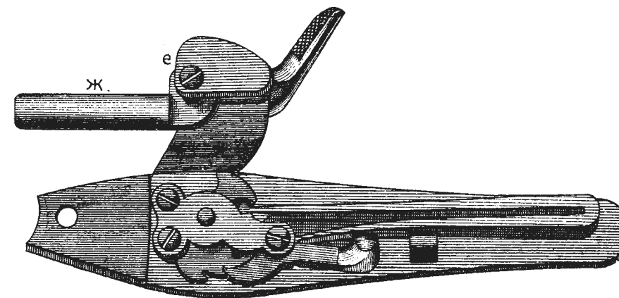
Рис.137. Замокъ.
