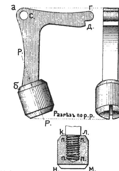
Рис.208. Спускъ казачій.
