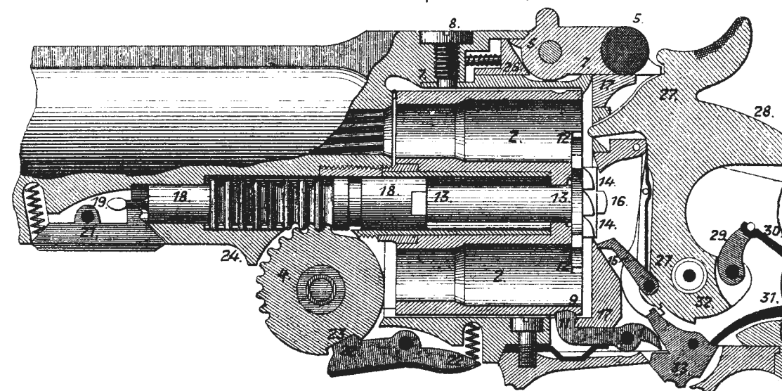
Рис.270. Револьверъ закрытъ.
