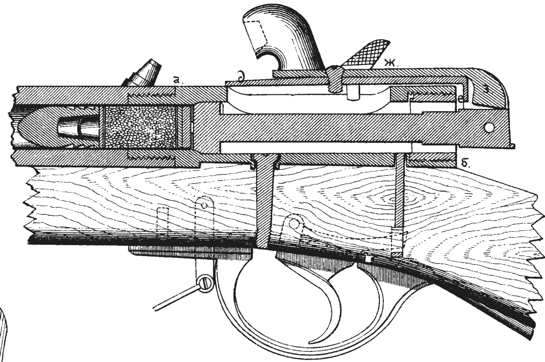
Рис.82. Продольный разрезъ.
