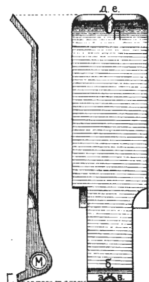
Рис. 113. Длинная прицѣльн. рамка.
