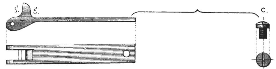
Рис.191. Спусковая пружина.
