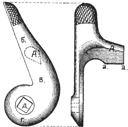
Рис.154.Курокъ.
