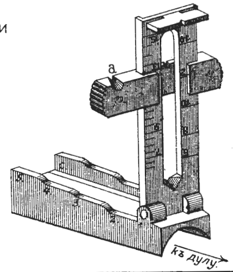
Рис.218.Боковой прицѣль.
