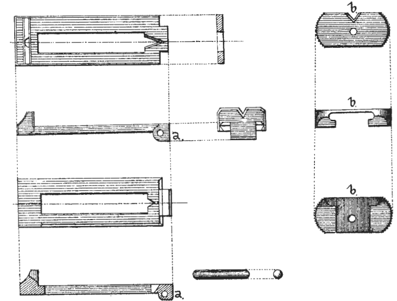
Рис.183. Прицѣль.
