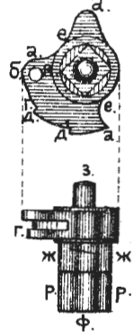
Рис.155.Ладыжка.
