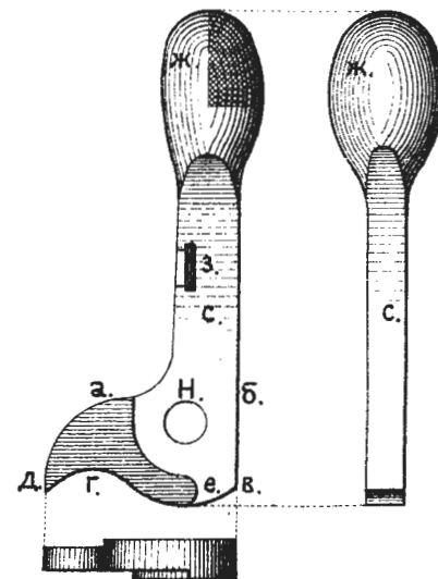
Рис. 99. Рукоятка.
