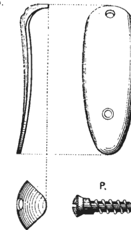
Рис.250. Затылок драгунск. винтовки.
