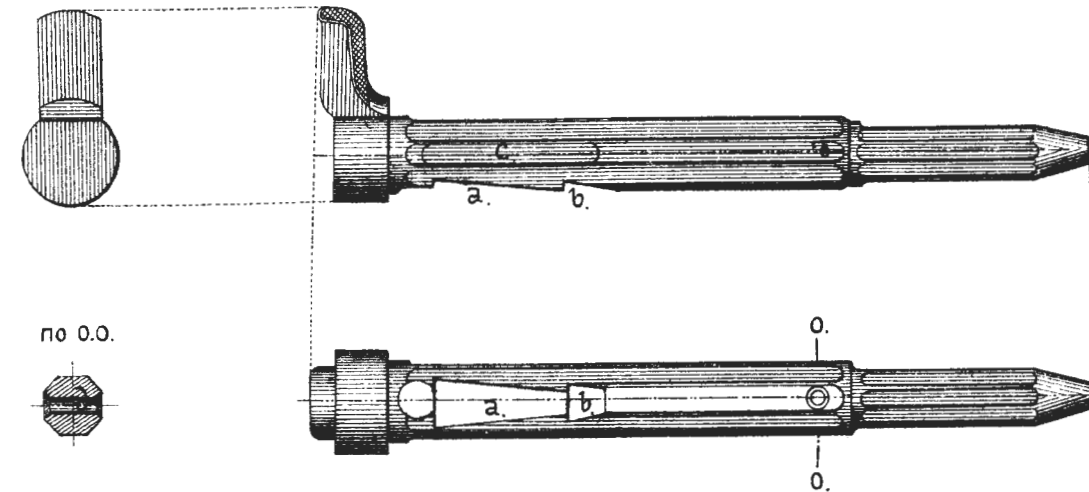
Рис.187. Курокъ.
