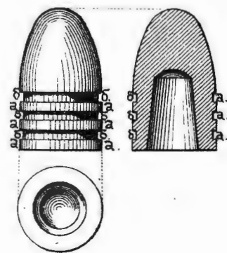
Рис.167. Пуля.
