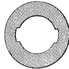
Рис. 5. Поперечное сечение ствола двухнарезного штуцера.
