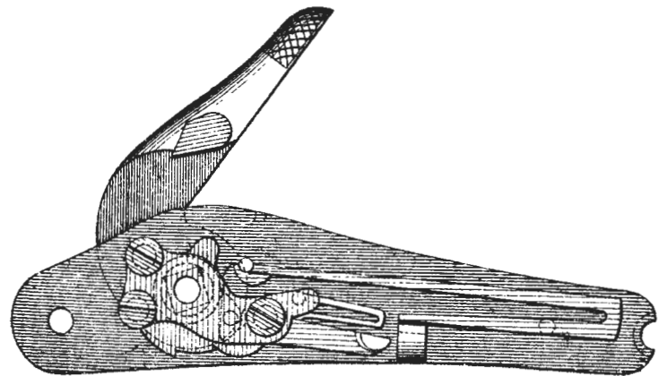
Рис.152.Замокъ въ собран. видѣ.
