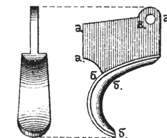
Рис. 110. Спускъ.
