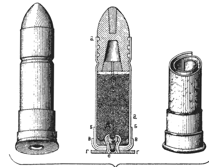
Рис. 74. Составной металлическій патронъ Боксера.
