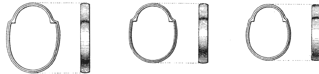
Рис.251. Глухия кольца казачьей винтовки. нижнее. среднее. верхнее.
