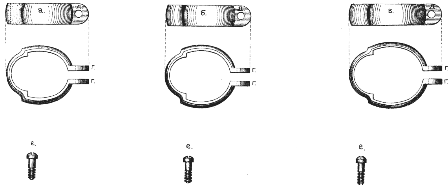
Рис.121. Ложевыя кольца.
