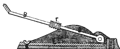
Рис.274. Прицѣль къ кръпостному ружью.
