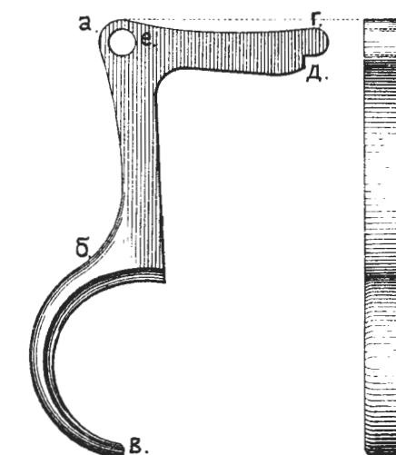
Рис.207. Спускъ драгунскій.
