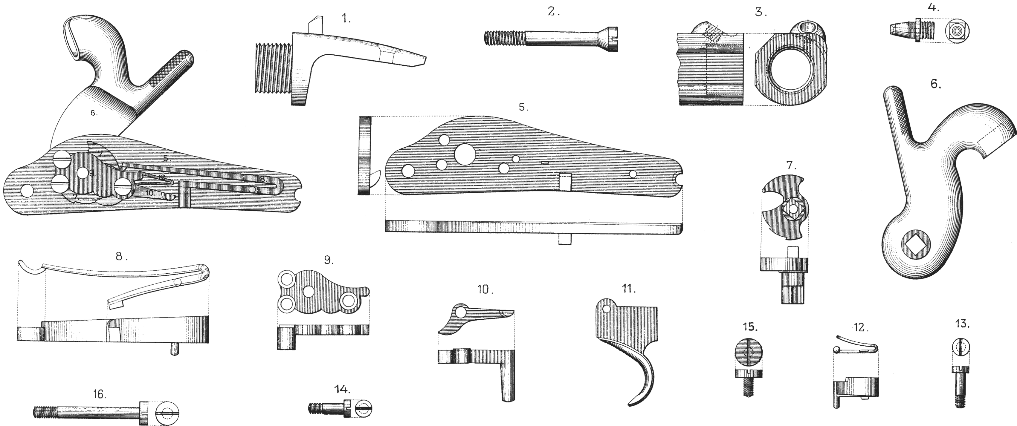
Рис.36. Части ударного пьхотного ружья обр.1845г.
