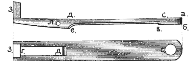
Рис. 92. Пружина.
