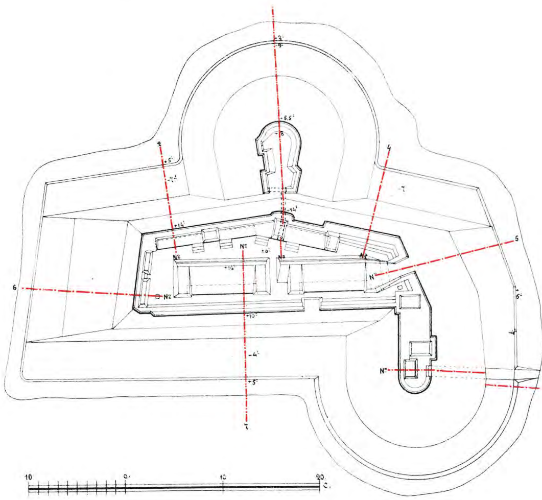
Планъ форта № I.
