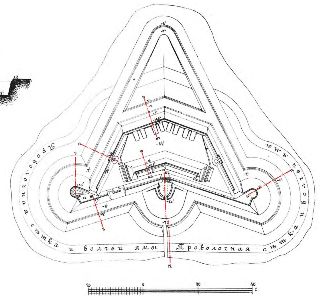
Планъ форта № IV.
