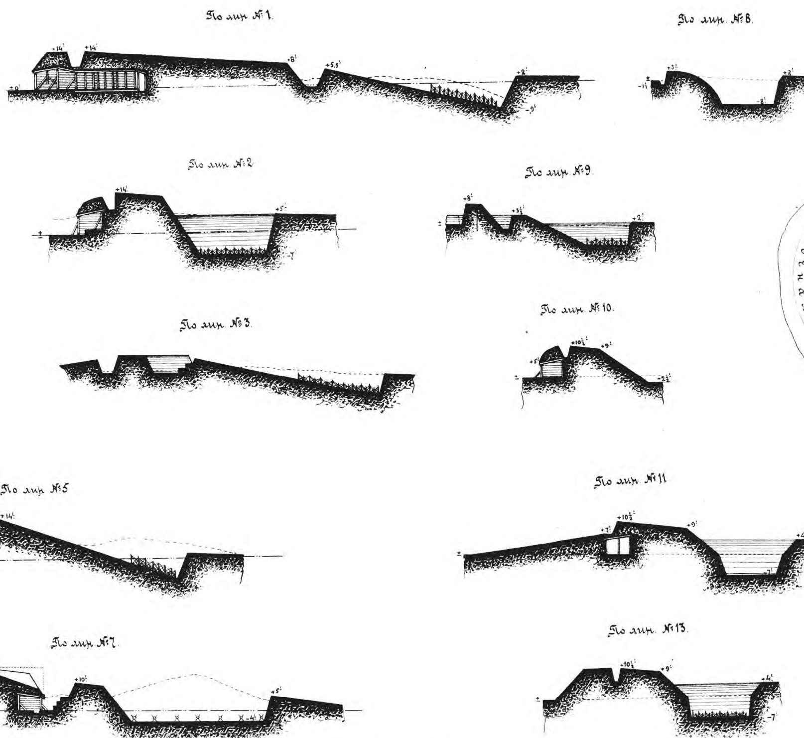
Профили къ планамъ фортовъ
